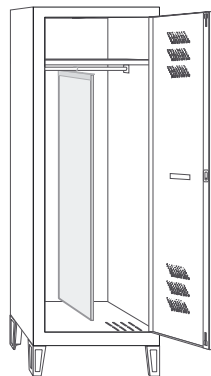
10 Hängende PVC-Trennwand Nr. 536490
