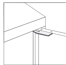
11 Türanschlag für Türen in Bolzen gelagert, max. Türöffnung 110° Nr. 500090
